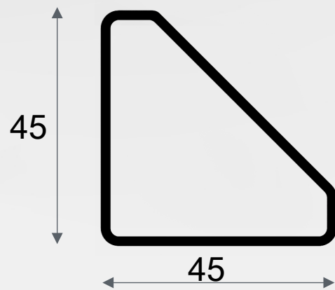
PERFIL LINEA PRISMA LIGHT
